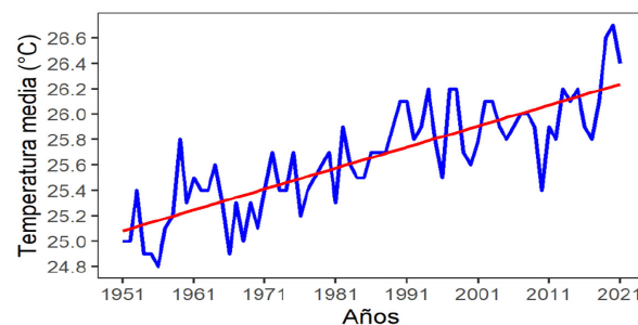
Figura 4. Temperatura media anual en Cuba durante el período 1951-2021. La línea roja representa la tendencia lineal.
