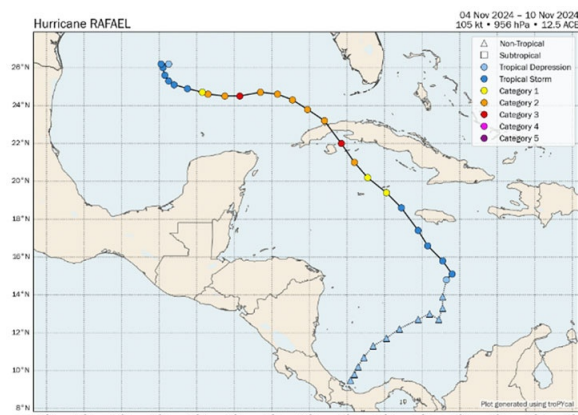
Figura 24. Trayectoria del huracán Rafael.
