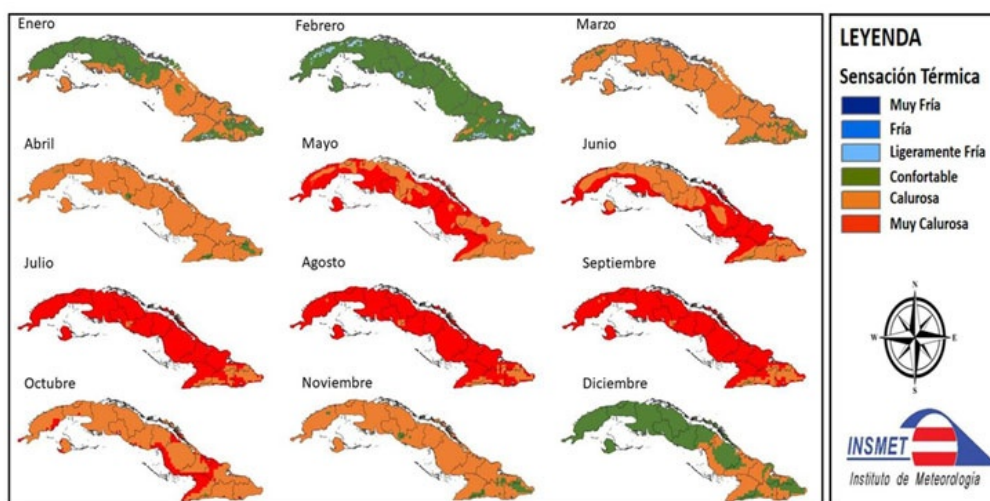
Figura 10. Sensación térmica media a la 1:00 pm determinada a partir de la Temperatura Efectiva (TE) durante el 2024.
