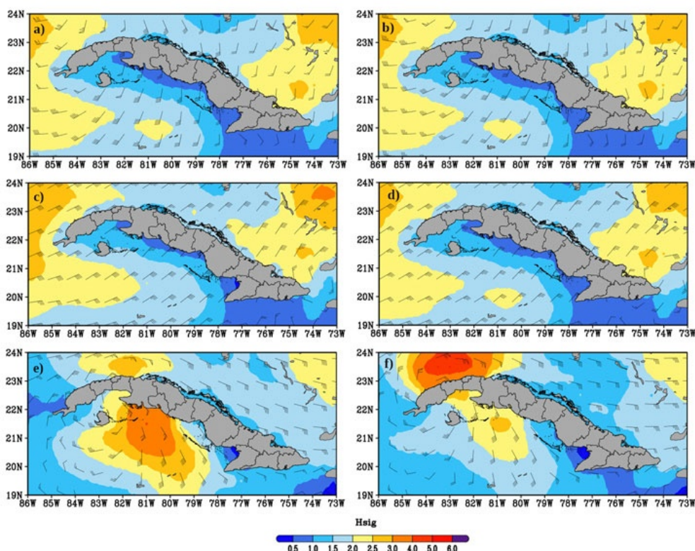
Figura 6. Velocidad y dirección del viento (barbas) en km/h y Hsig (m) en las costas cubanas al paso de los huracanes Milton, Oscar y Rafael. a) 9 oct 2024-12Z, b) 9 oct.2024-18Z, c) 20 oct 2024-12Z d) 20 oct 2024-18Z, e) 6 nov 2024-18Z y f) 7 nov 2024-00Z.
