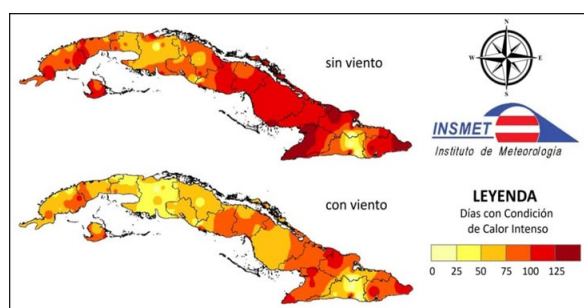
Figura 11. Cantidad de días con Condición de Calor Intenso (CCI) durante el 2024.
