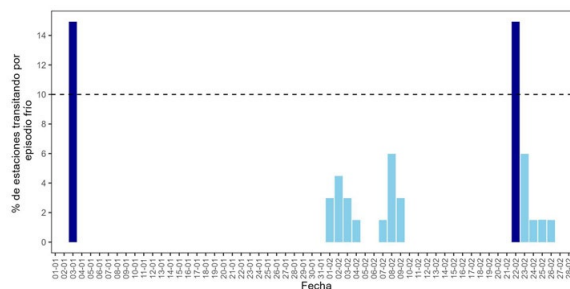
Figura 17. Porcentaje de estaciones meteorológicas de Cuba transitando por un episodio frío según la variante 3. En azul oscuro cuando superan el 10% de estaciones
