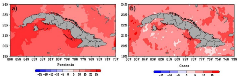
Figura 14. Indicadores extremos climáticos para áreas oceánicas referidos a Hsig durante el años 2024 respecto al periodo de referencia 1991-2020, a) HsigFD y b) HsigCD.
