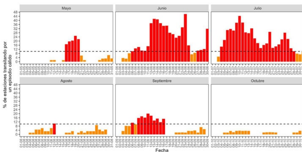
Figura 15. Porcentaje de estaciones meteorológicas de Cuba transitando por un episodio cálido según la variante 2. En rojo cuando superan el 10%. Se presentaron cinco eventos extremos por calor y varios días cálidos.
