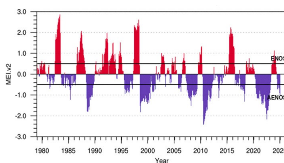
Figura 2. Índice multivariado (MEI) de El Niño/Oscilación del Sur (ENSO).
