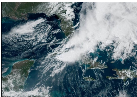
Figura 3. Imagen del satélite GOES-16 del día 23 de marzo de 2024.
