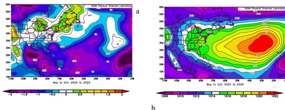
Figura 1. Anomalías (a) y presión atmosférica (b) de presión a nivel del mar.
