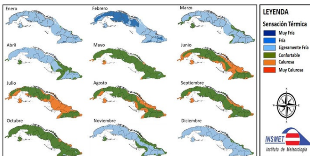
Figura 9. Sensación térmica media a la 7:00 am determinada a partir de la Temperatura Efectiva (TE) durante el 2024.
