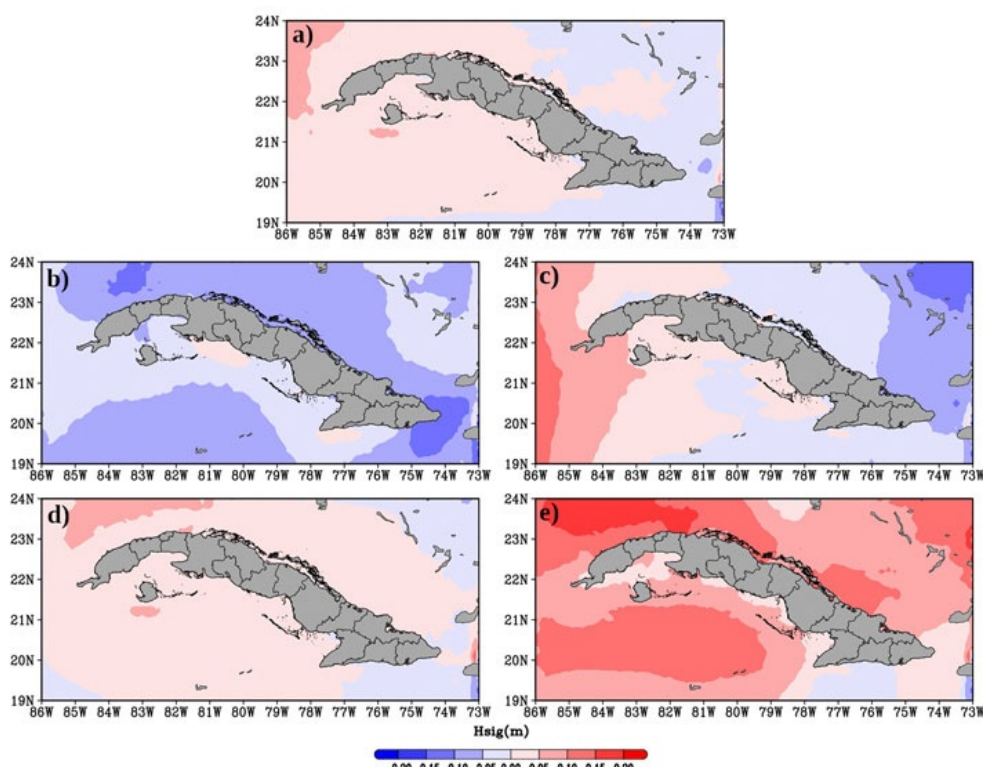
Figura 5. Anomalías de Hsig durante el año 2024 respecto a la norma climática 1991-2020. a) anual, b) enero-marzo, c) abril-junio, d) julio-septiembre y e) octubre-diciembre.
