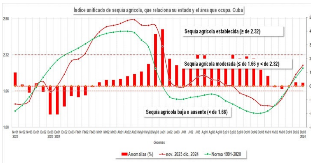
Figura 21. Índice unificado de sequía agrícola para Cuba (relaciona su estado y el área que ocupa, así como valores de su anomalía).
