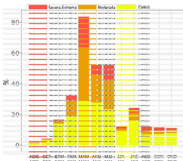
Figura 20. Marcha trimestral del por ciento de área en Cuba afectada por sequía meteorológica.
