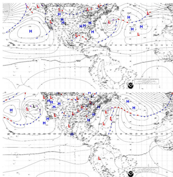
Figura 18. Mapa sinóptico de superficie del 03/01/2023 (a) 22/02/2024 (b) (12 UTC). Cuba se encuentra bajo la influencia de un anticiclón continental migratorio.
