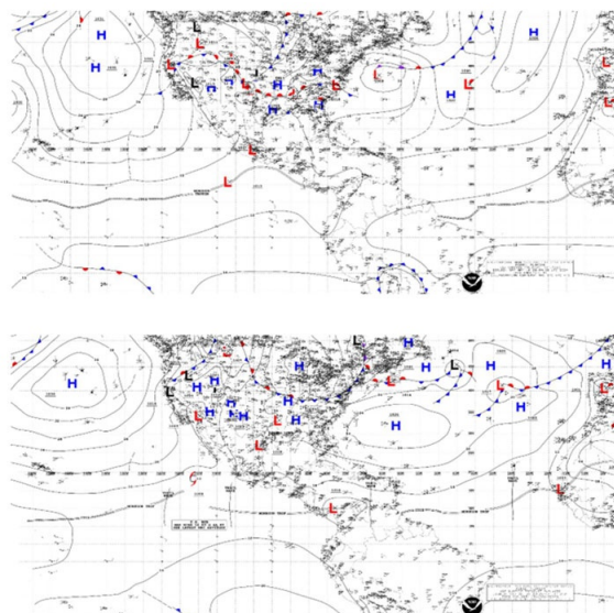
Figura 16. Mapa sinóptico de superficie del 18/05/2024 (a) y 25/07/2024 (b) (18 UTC). Extraído de, https://ftp.nhc.ncep.noaa.gov/tafb/surface_analysis/2024/ .
