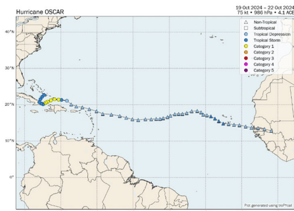
Figura 23. Trayectoria del huracán
