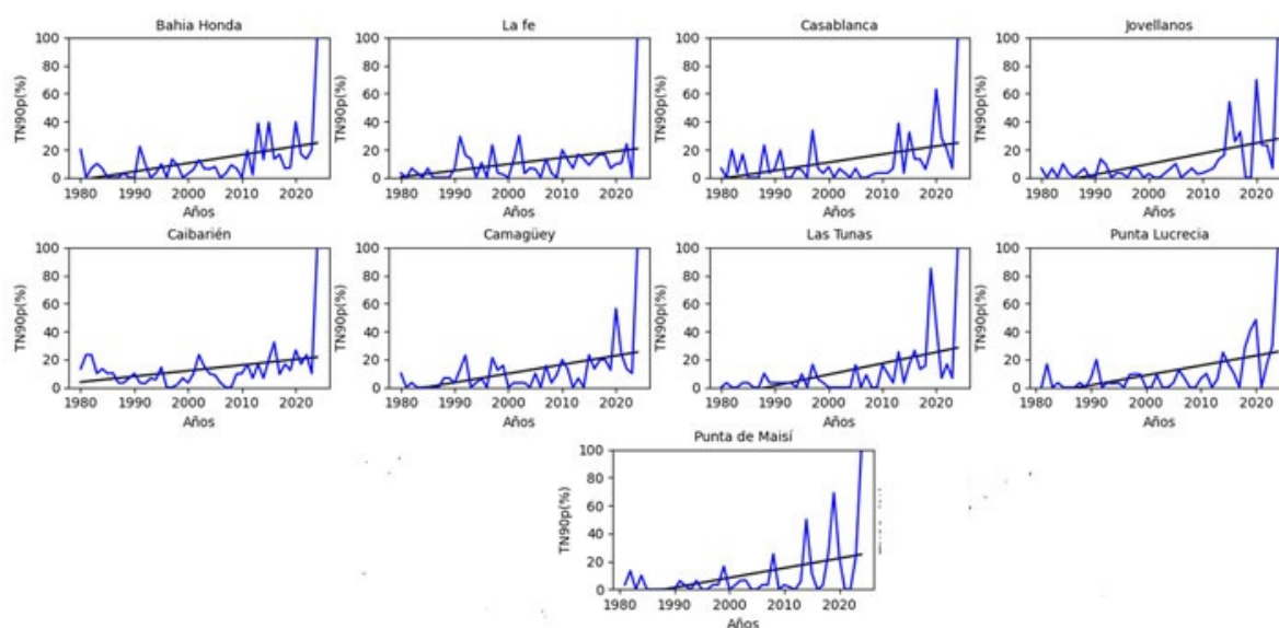
Figura 13. Por ciento de noches cálidas en el mes de Abril durante el periodo 1980-2024. Norma 1991-2020.
