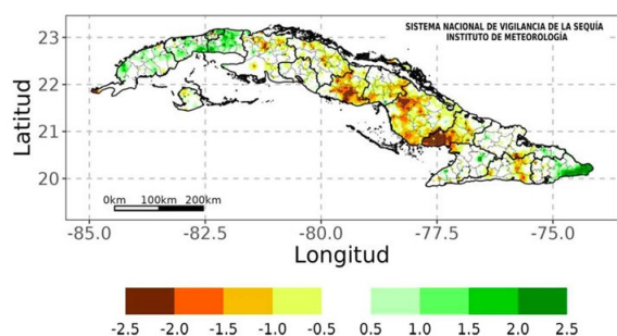
Figura 8. Distribución espacial de los acumulados de precipitación durante el período enero-diciembre de 2024, expresados según el índice de precipitación estandarizada (SPI12).
