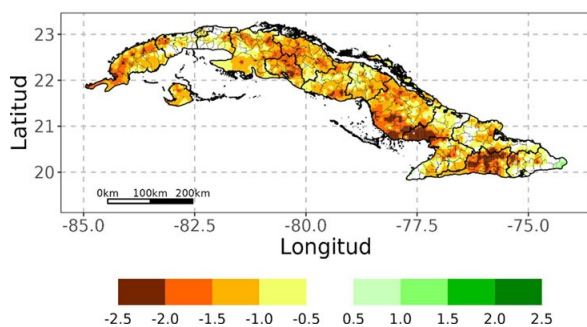
Figura 19. Distribución espacial de los acumulados de precipitación durante el período marzo-mayo de 2024, expresados según el índice de precipitación estandarizada (SPI3)
