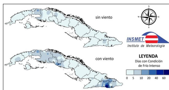
Figura 12. Cantidad de días con Condición de Frío Intenso (CFI) durante el 2024.
