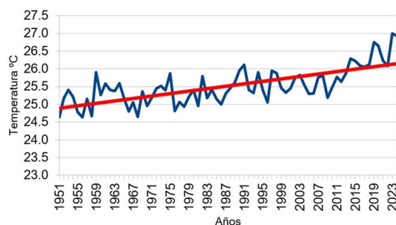
Figura 7. Temperatura media anual en Cuba durante el período 1951-2024. La línea roja representa la tendencia lineal.
