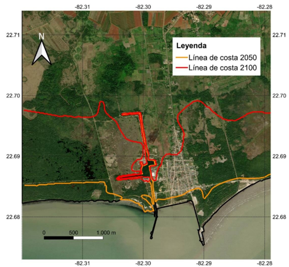
Figura 4. Líneas de costa para los escenarios de 2050 y 2100
