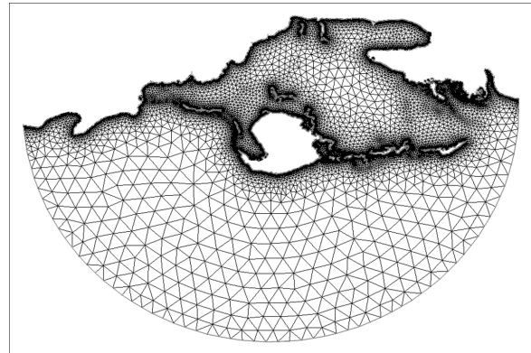
Figura 3. Malla utilizada para la simulación con ADCIRC+SWAN
