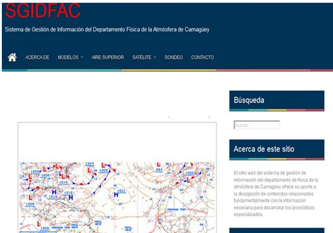
Figura 8. Mapa del tiempo en superficie
