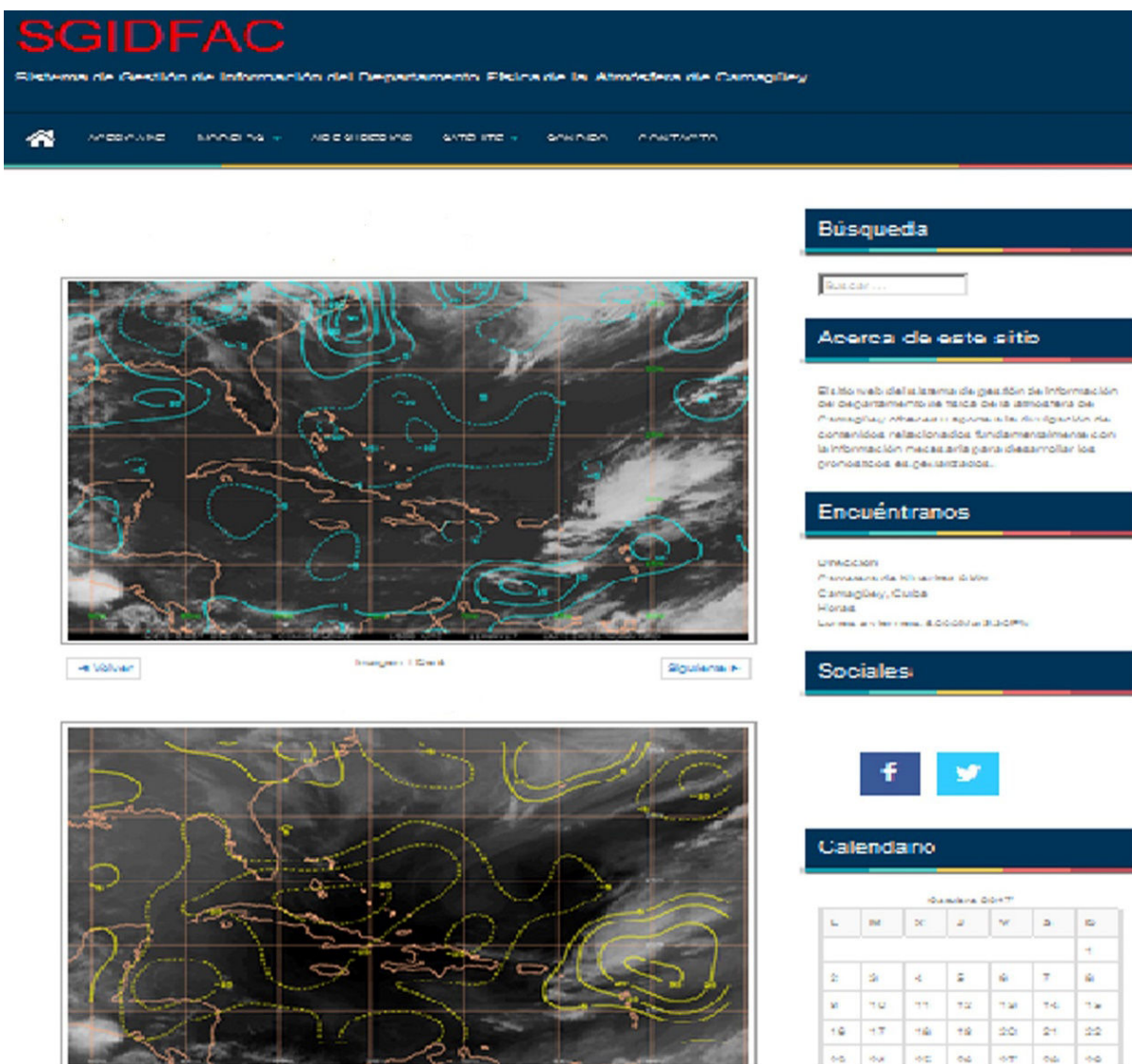
Figura 9. Análisis de la convergencia y divergencia.
