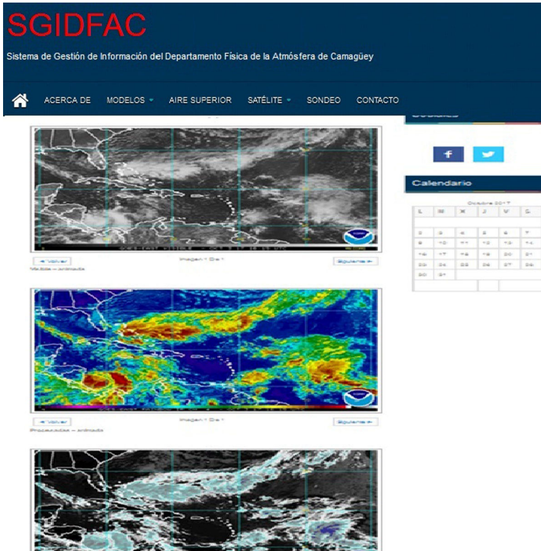
Figura 13. Imágenes visibles e infrarrojas de satélite
