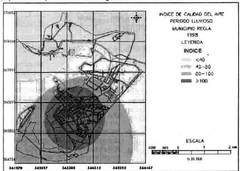
Figura4. Índice de Calidad del Aire calculado para el municipio de Regla (año 1998)
