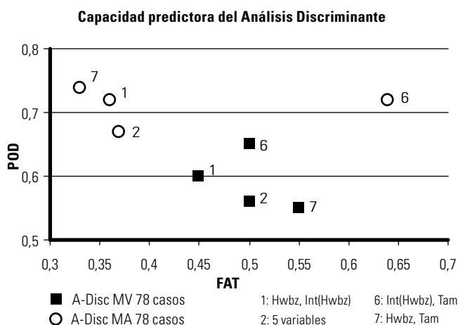
Fig. 3. Capacidad de predicción de algunas pruebas del análisis discriminante.
