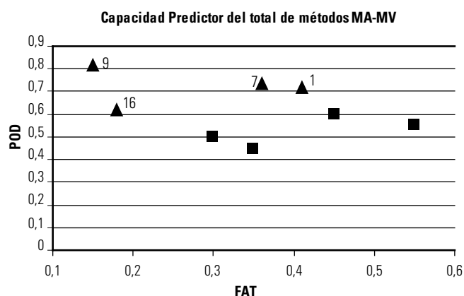
Fig. 5. Capacidad de predicción total de los dos métodos.
