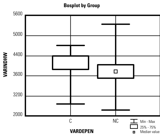
Fig. 1. Diagrama de la altura de la isoterma de 0 °C del bulbo húmedo (eje ordenadas, en metros) para los dos grupos de clasificación (C/NC ocurrencia/no ocurrencia de granizos respectivamente).
