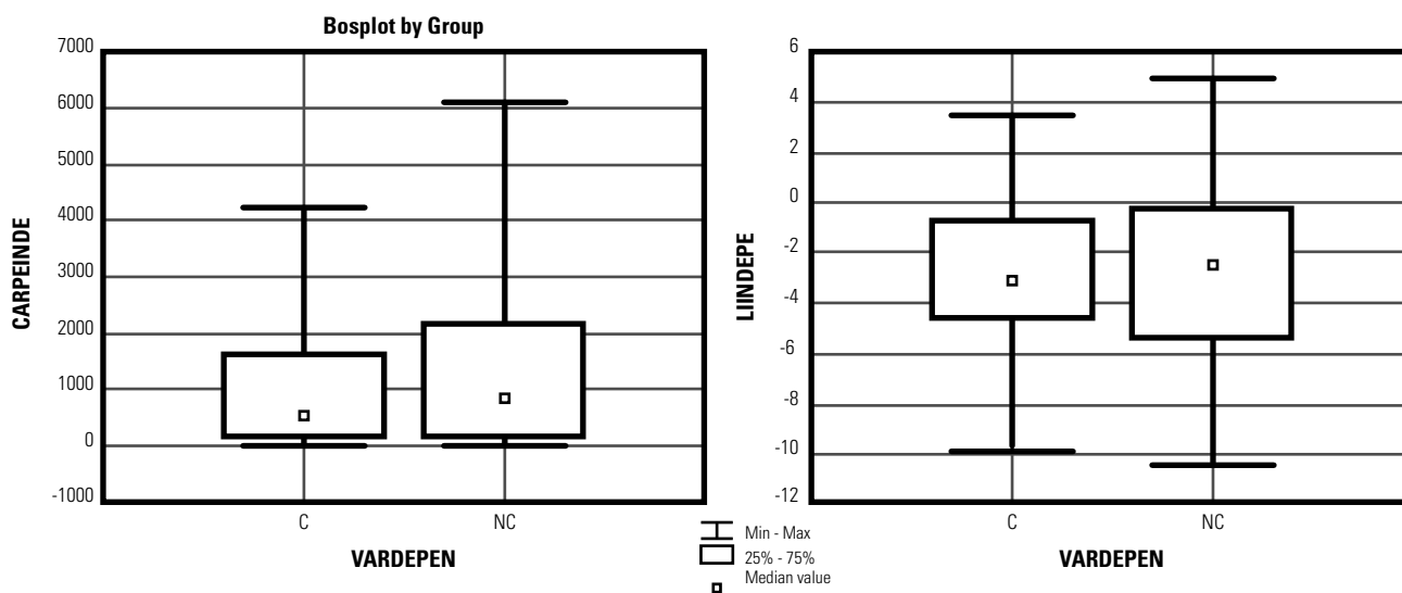
Fig. 2. Diagrama de las variables CAPE (J/Kg) y LI, para los dos grupos de clasificación.
