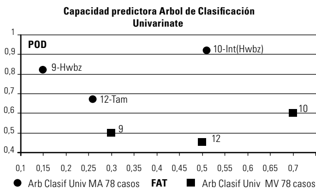
Fig. 4. Capacidad de predicción de las pruebas univariantes de los árboles de clasificación.
